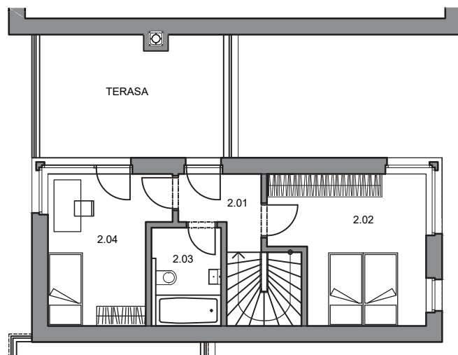
PŮDORYS 2.N.P.
